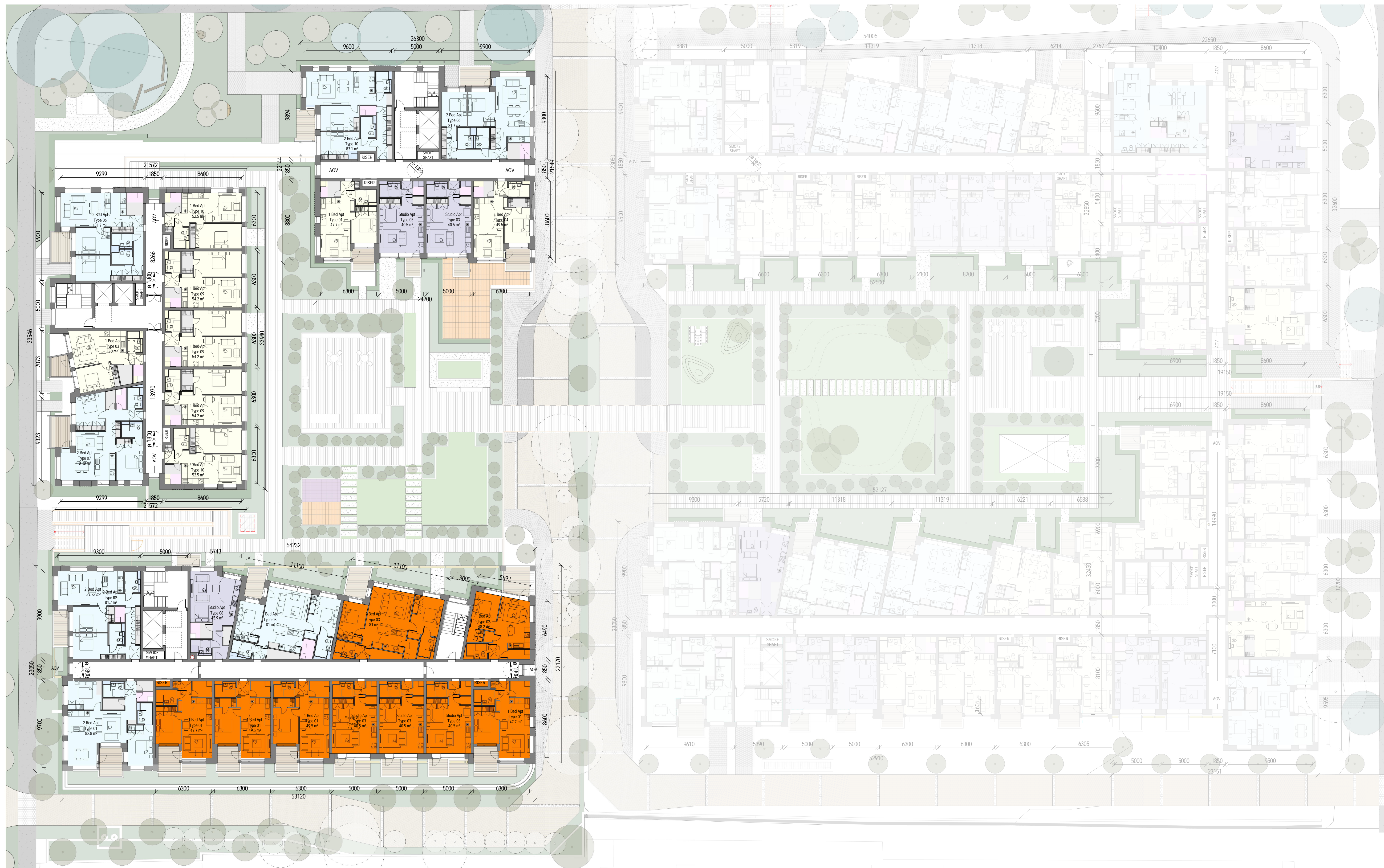
1 01 FLOOR - PART V - TACK SITE 90012 1 : 200
